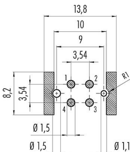
Leiterplattenlayout
