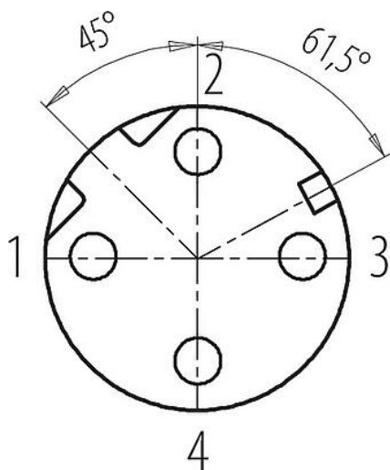
Polbild (Steckseite)
