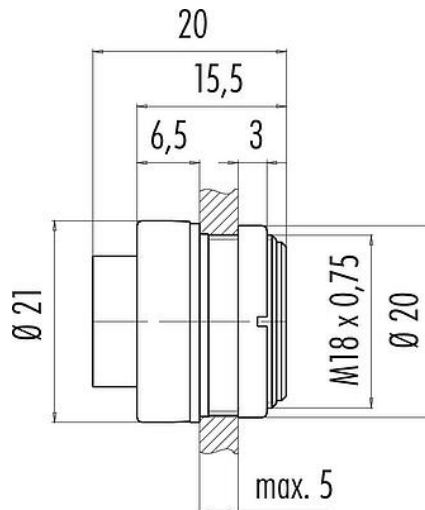
Maßzeichnung
