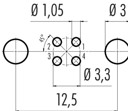
Leiterplattenlayout
