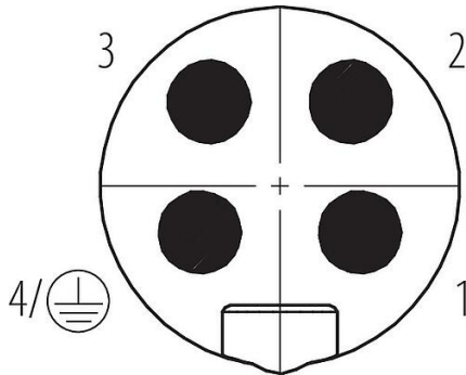
Polbild (Steckseite)
