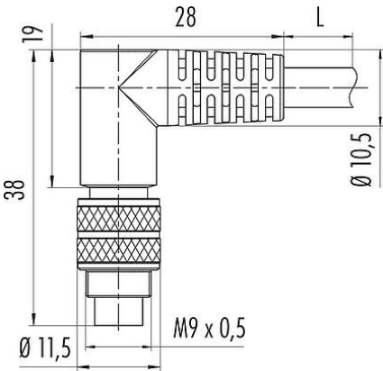
Maßzeichnung
