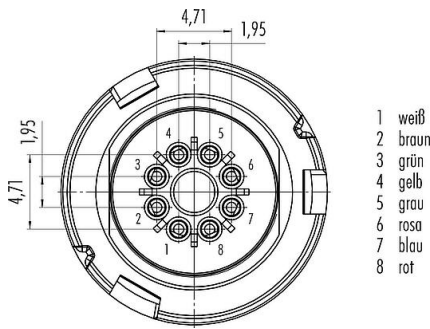
Polbild (Steckseite)
