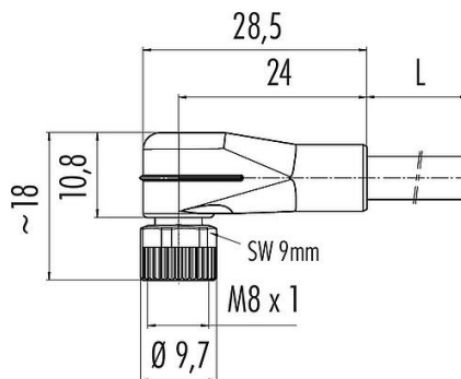
Maßzeichnung
