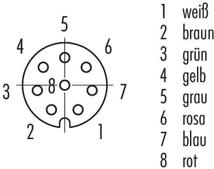
Polbild (Steckseite)
