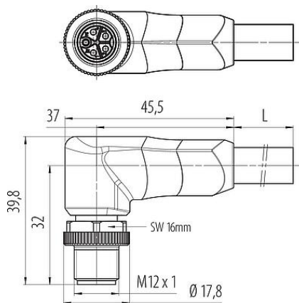
Maßzeichnung
