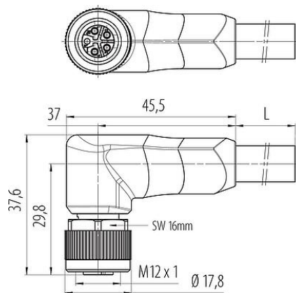
Maßzeichnung
