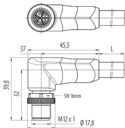
Maßzeichnung
