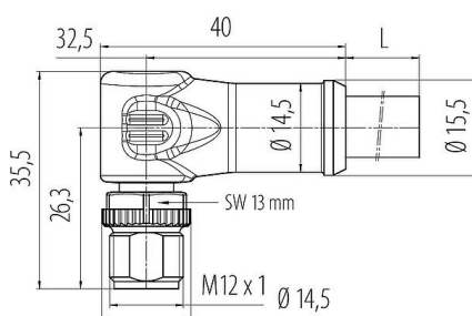
Maßzeichnung
