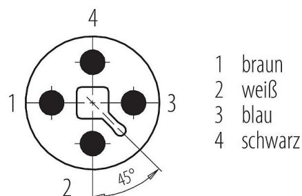
Polbild (Steckseite)
