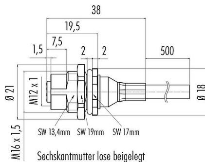
Maßzeichnung
