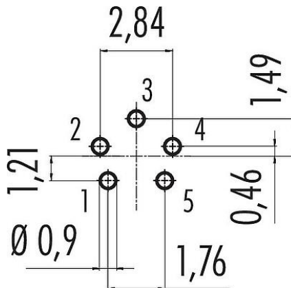
Leiterplattenlayout
