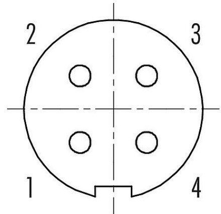
Polbild (Steckseite)
