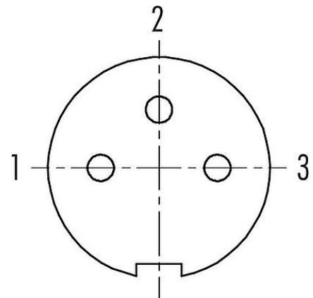
Polbild (Steckseite)
