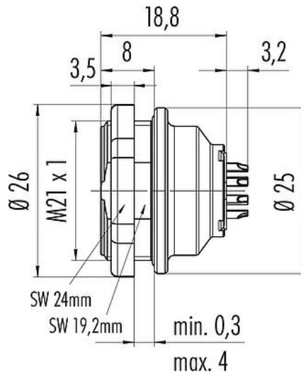
Maßzeichnung
