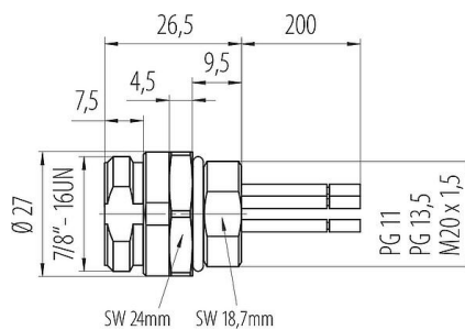
Maßzeichnung
