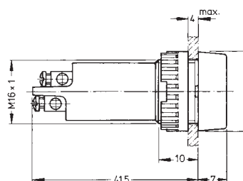
Schraubanschluss
