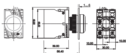
mit Schaltelement
