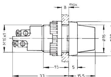
Schraubanschluss
