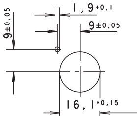
Einbauöffnung
