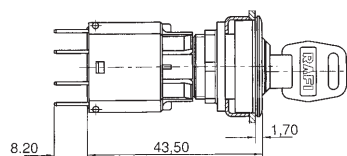
Schaltelement Steckanschluss mit RAFIX 16 F Schlüsselschalter
