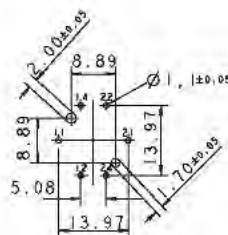
Lochbild Leiterplatte, Bauteilseite
