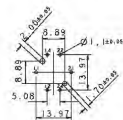
Lochbild Leiterplatte, Bauteilseite
