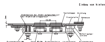
Einbau von hinten
