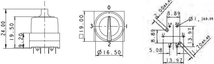
Lochbild Leiterplatte, Bauteilseite
