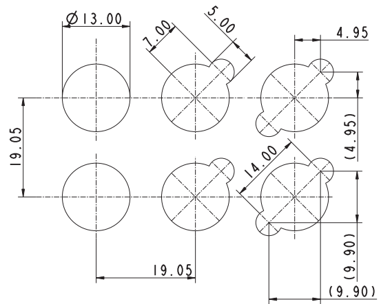
RF 15 R, beleuchtet
