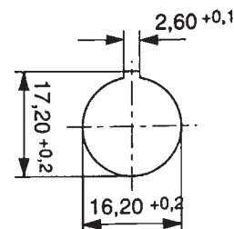
Einbauöffnung
