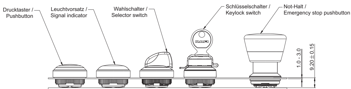
Maßzeichnung RAFX 22 FSR, PCB
