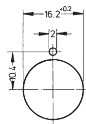
Einbauöffnung
