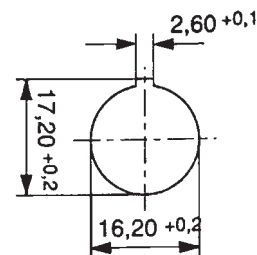
Einbauöffnung
