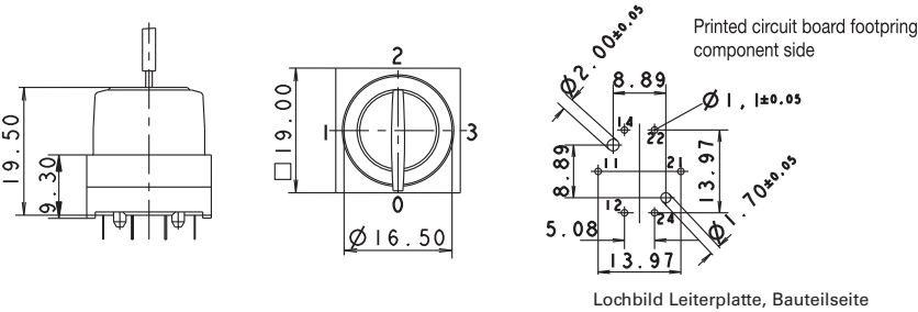
Lochbild Leiterplatte, Bauteilseite
