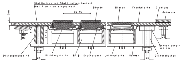
Einbau von vorne
