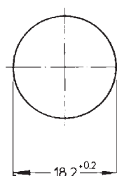
Einbaubohrung
