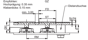
SMT-Gullwing-Anschluss
