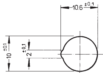
Einbauöffnung
