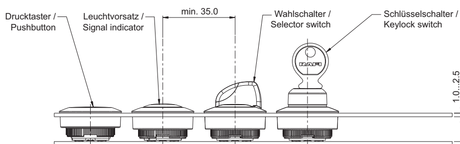
Maßzeichnung RAFX 30 FS + , PCB
