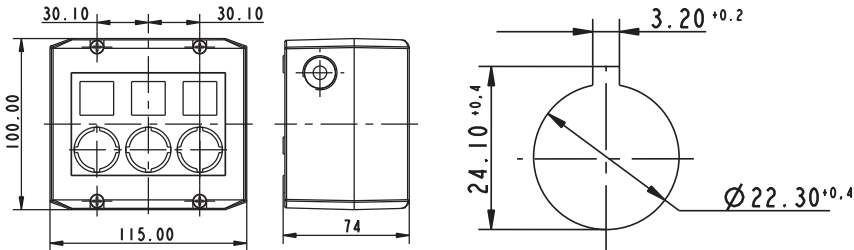
Einbauöffnung nach IEC 60947-5-1
