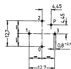
Leiterplatten-Bohrbild, Sicht auf Bauteilseite
