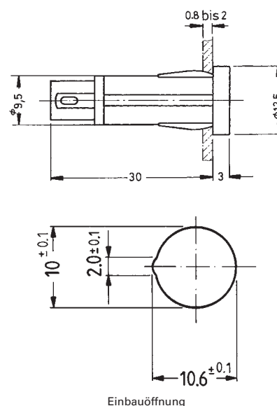
Einbauöffnung
