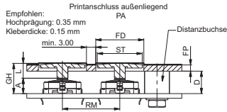
THT-Anschluss außenliegend
