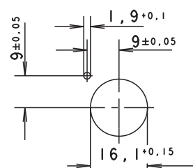
Einbauöffnung
