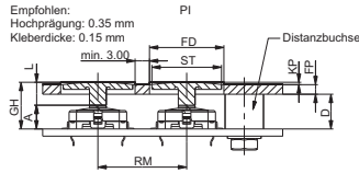
THT-Anschluss innenliegend
