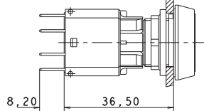
Schaltelement Steckanschluss mit RAFIX 16 Drucktaster
