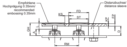
THT-Anschluss außenliegend
