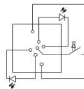
Taster Vollausleuchtung
