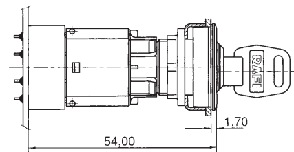
mit Leiterplattenstecksockel
