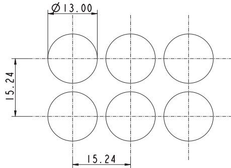
RF 15 R, unbeleuchtet
