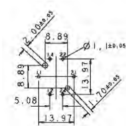
Lochbild Leiterplatte, Bauteilseite
