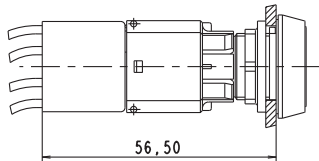
... mit Gruppenanschlussstecker
