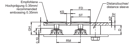
SMT-Gullwing-Anschluss
