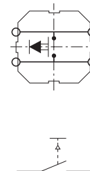
Schaltzeichen nach IEC 60 617 Form X (doppelt unterbrechend)
