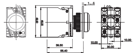
mit Schaltelement
