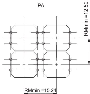
Sicht auf Bestückungsseite
