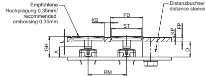
THT-Anschluss innenliegend
