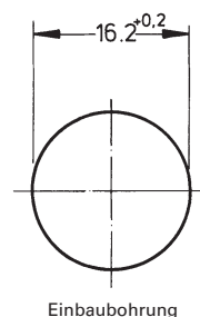
Einbaubohrung
