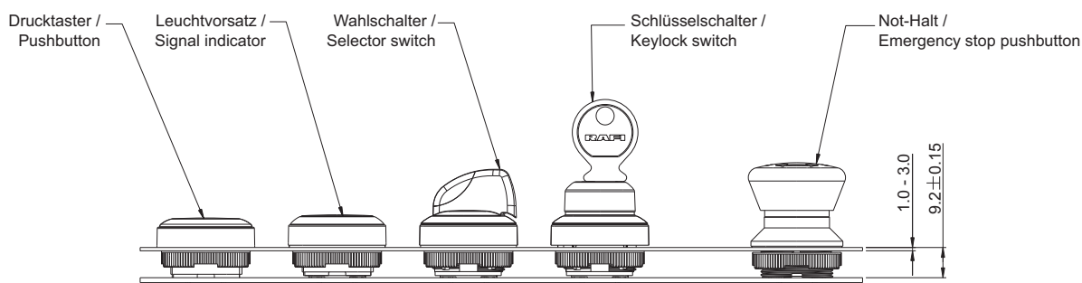
Maßzeichnung RAFX 22 FS + , PCB
