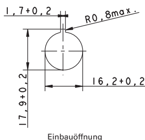
Einbauöffnung
