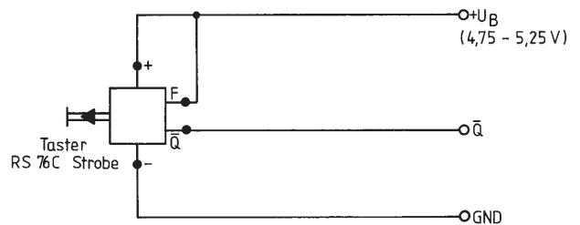
Verwendung als statischer Taster mit offenem Kollektorausgang. Ausgangstransistor (NPN) ist im betätigten Zustand leitend.
