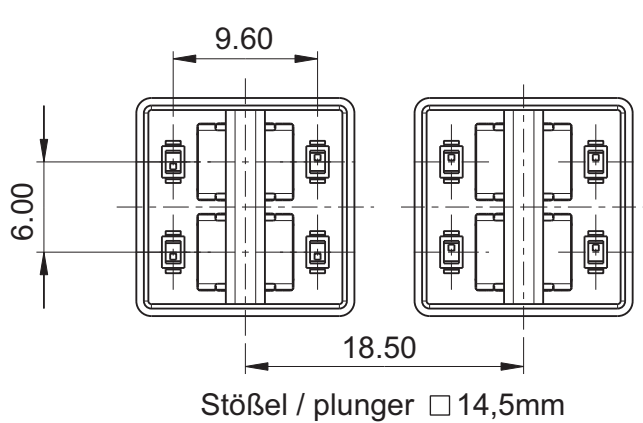
Stößel 14,5 x 14,5 mm
