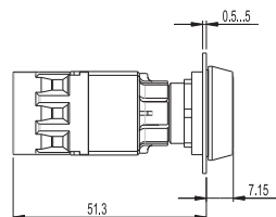
Schaltelement Schraubanschluss mit RAFIX 16 Drucktaster
