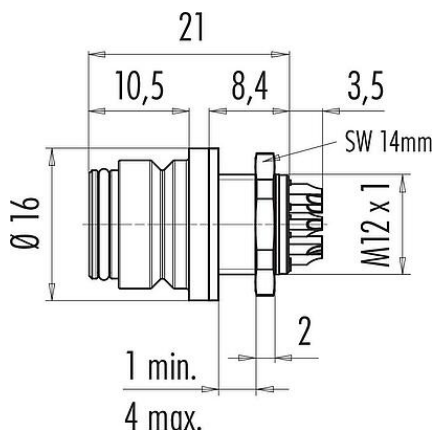
Maßzeichnung
