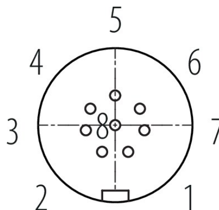
Polbild (Steckseite)
