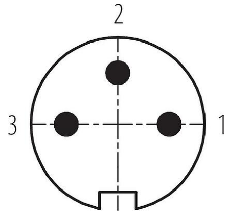
Polbild (Steckseite)
