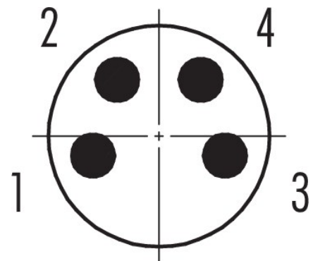
Polbild (Steckseite)
