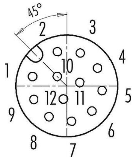
Polbild (Steckseite)
