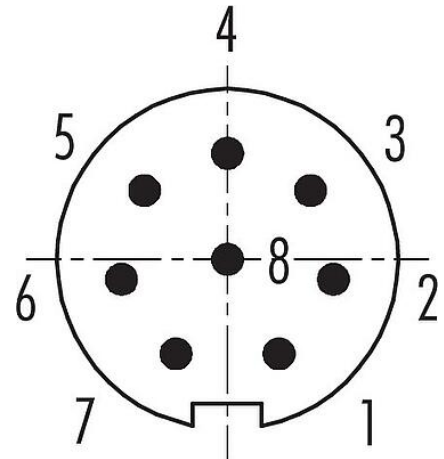
Polbild (Steckseite)
