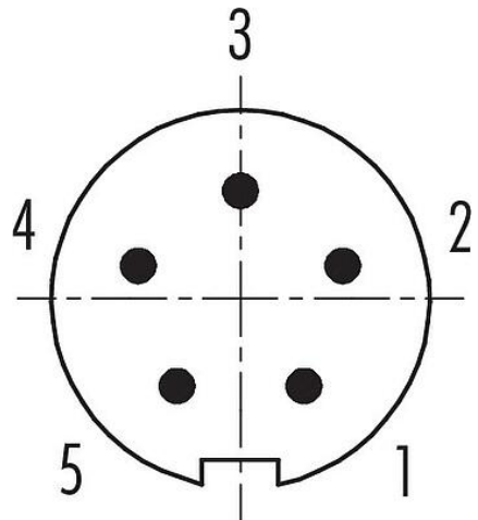
Polbild (Steckseite)
