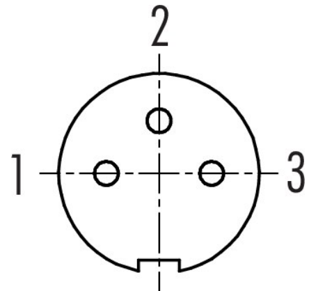
Polbild (Steckseite)
