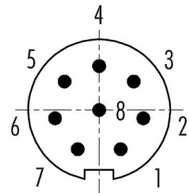
Polbild (Steckseite)
