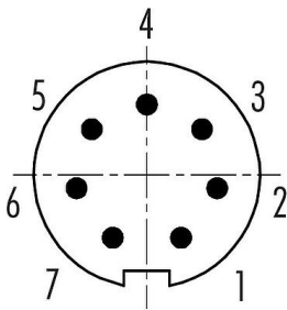
Polbild (Steckseite)
