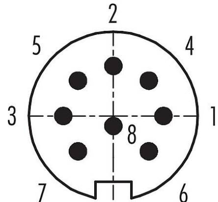
Polbild (Steckseite)
