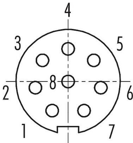
Polbild (Steckseite)
