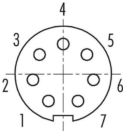
Polbild (Steckseite)
