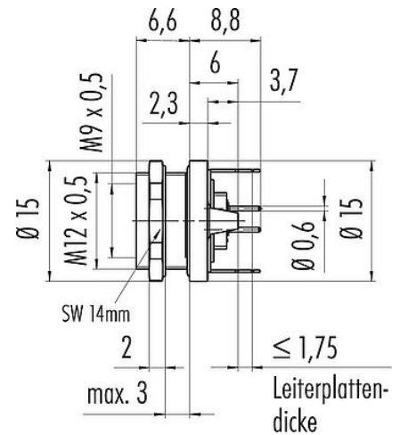
Maßzeichnung
