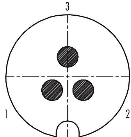
Polbild (Steckseite)
